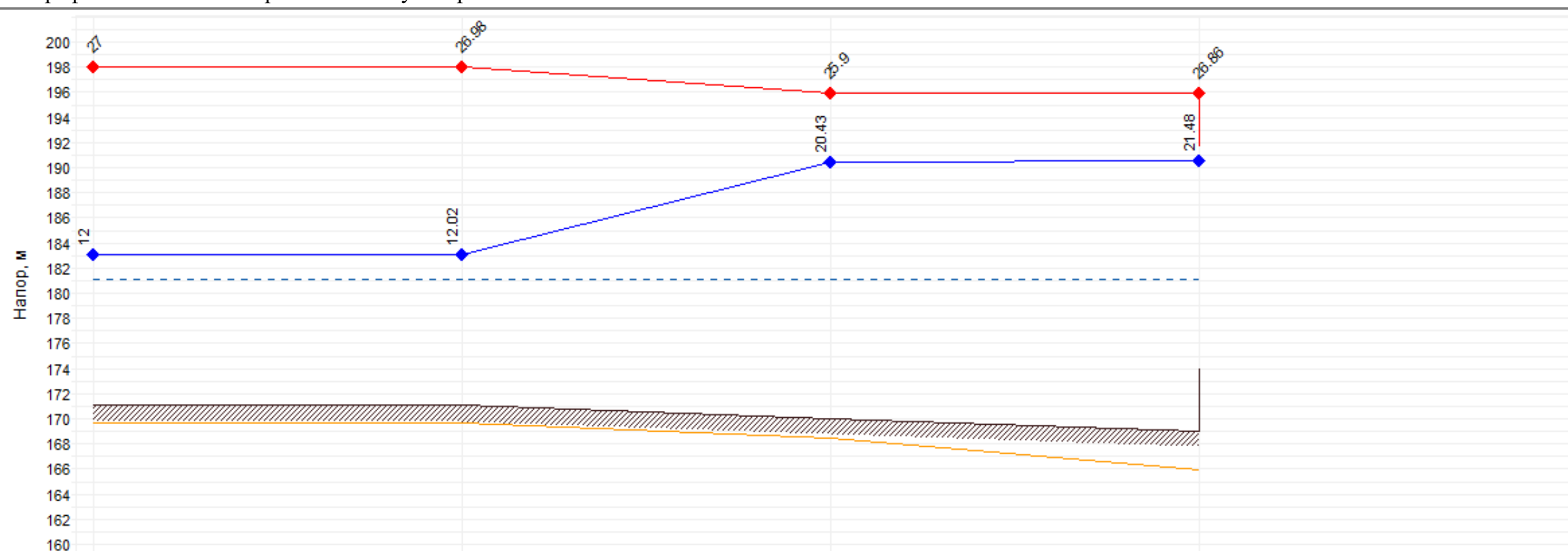
Пьезометрический график от котельной Врачебной амбулатории
