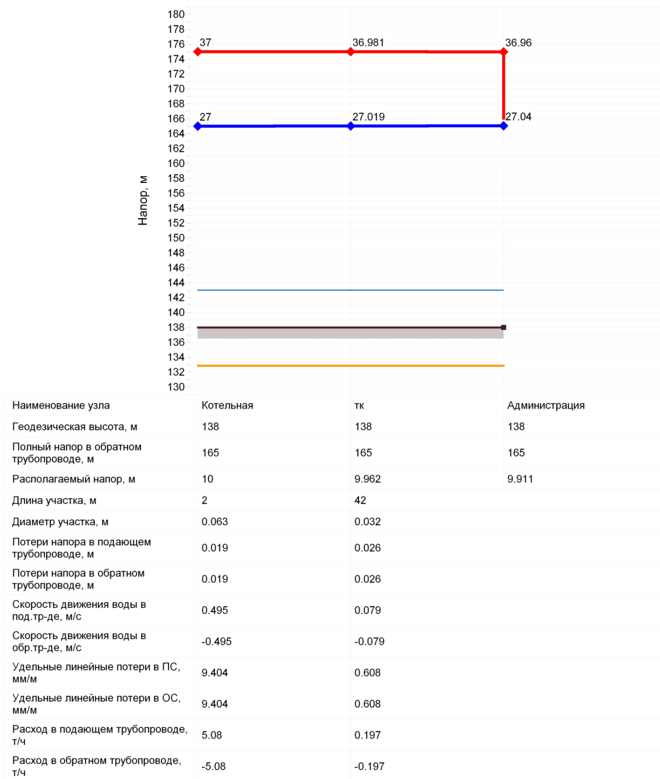
Рисунок 4 Пьезометрический график от котельной до Администрации, улица Советская, 14б.
