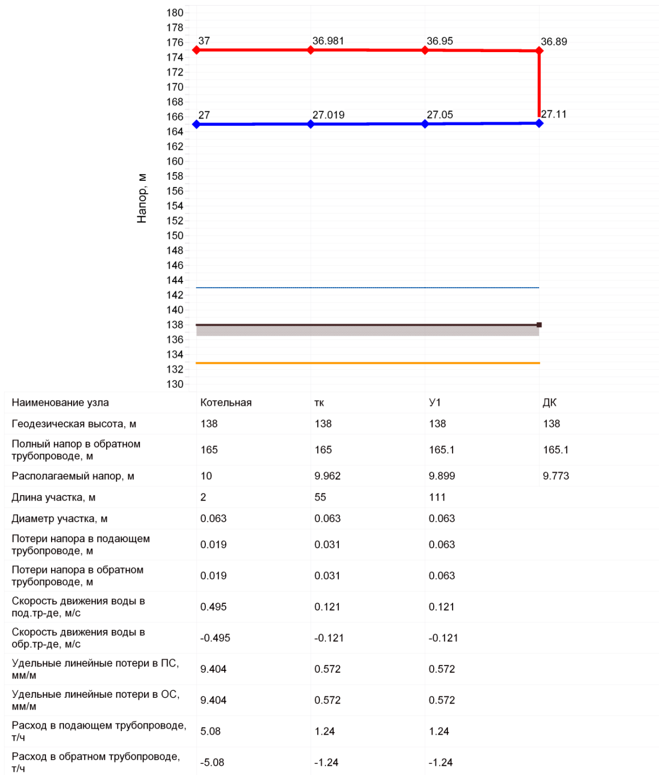
Рисунок 5 Пьезометрический график от котельной до СДК, улица Советская, 15а.
