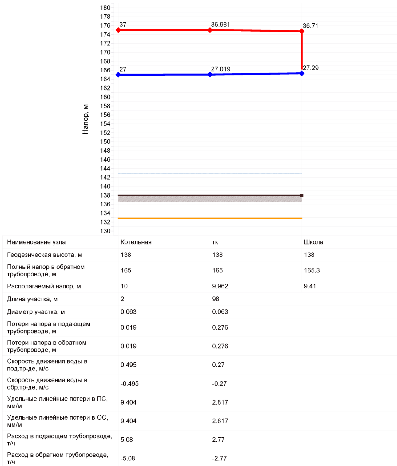
Рисунок 3 Пьезометрический график от котельной до Школы, улица Советская, 14в.
