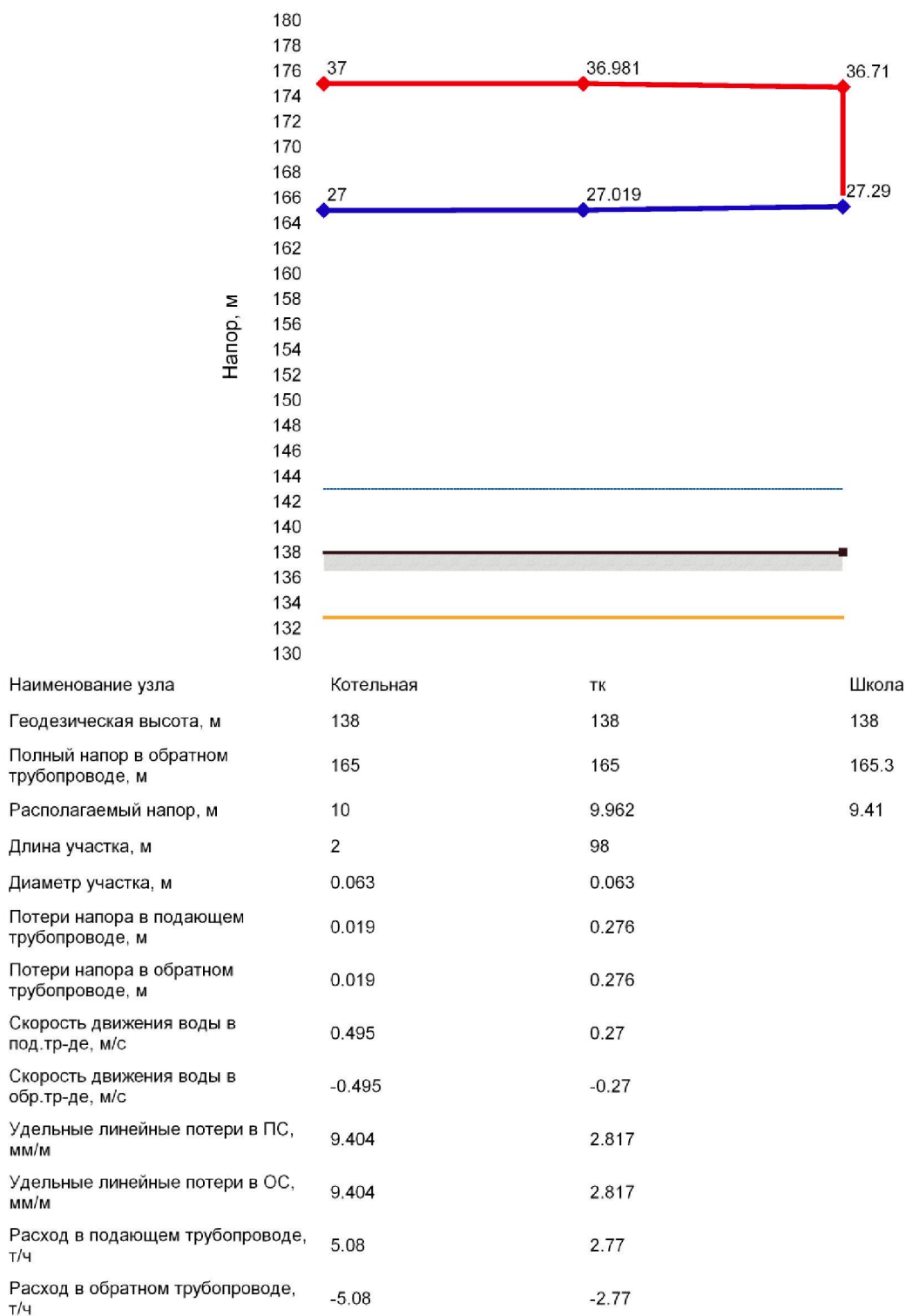
Рисунок 3 Пьезометрический график от котельной до Школы, улица Советская, 14в.
