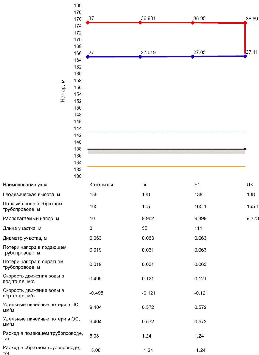
Рисунок 5 Пьезометрический график от котельной до СДК, улица Советская, 15а.
