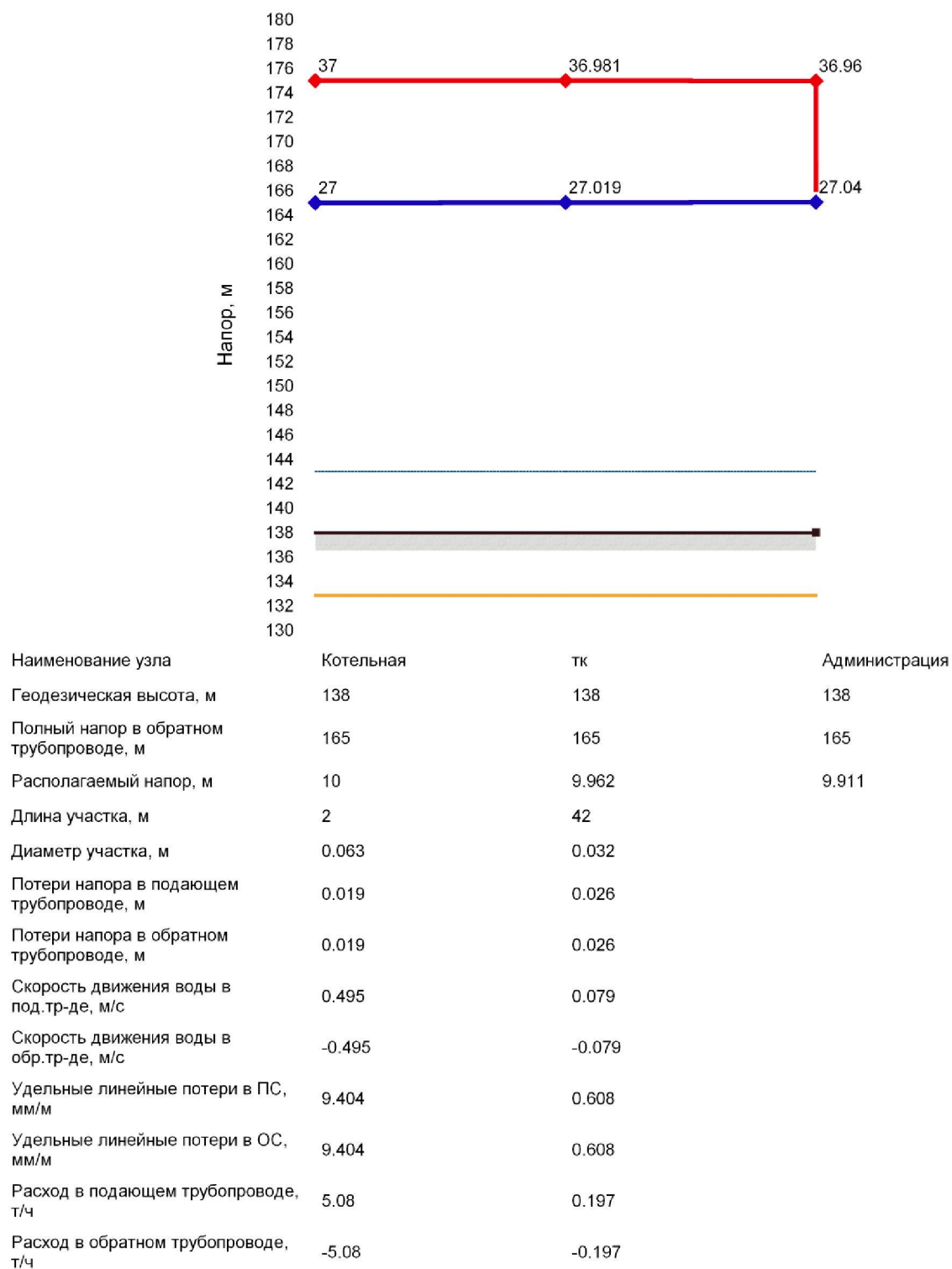
Рисунок 4 Пьезометрический график от котельной до Администрации, улица Советская, 14б.
