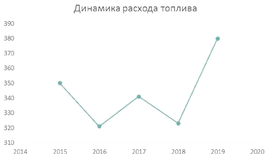
Рисунок 3 - Годовой расход угля на выработку тепловой энергии, тонн
