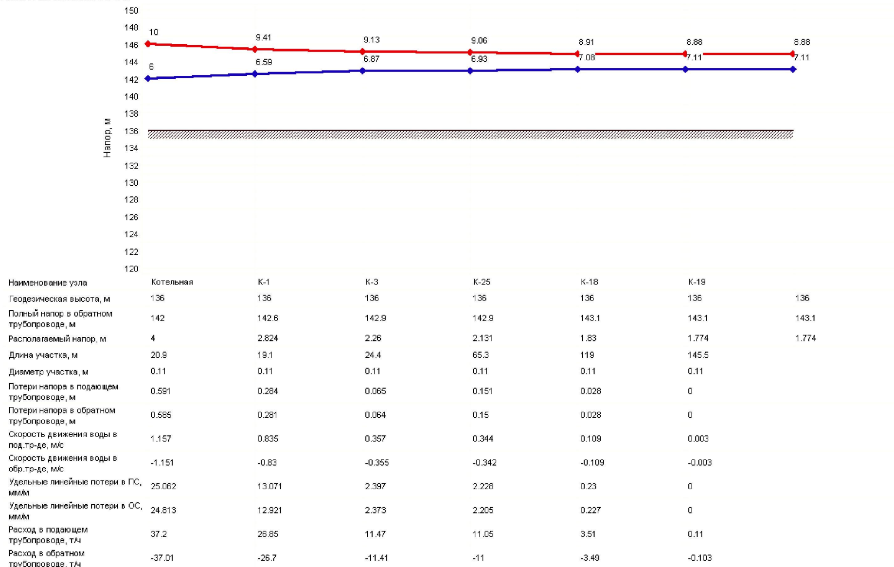
График от котельной до ул. Большевистская, 21
