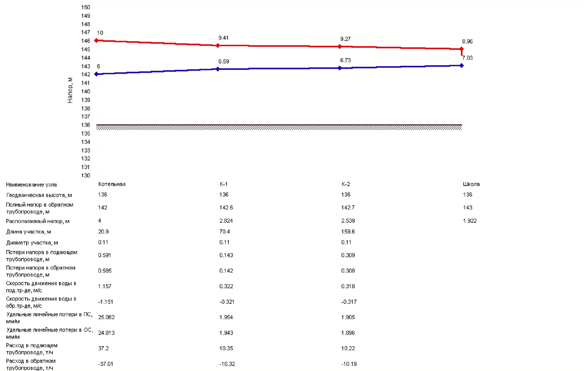
График от котельной до школы ул.Большевистская, 25
