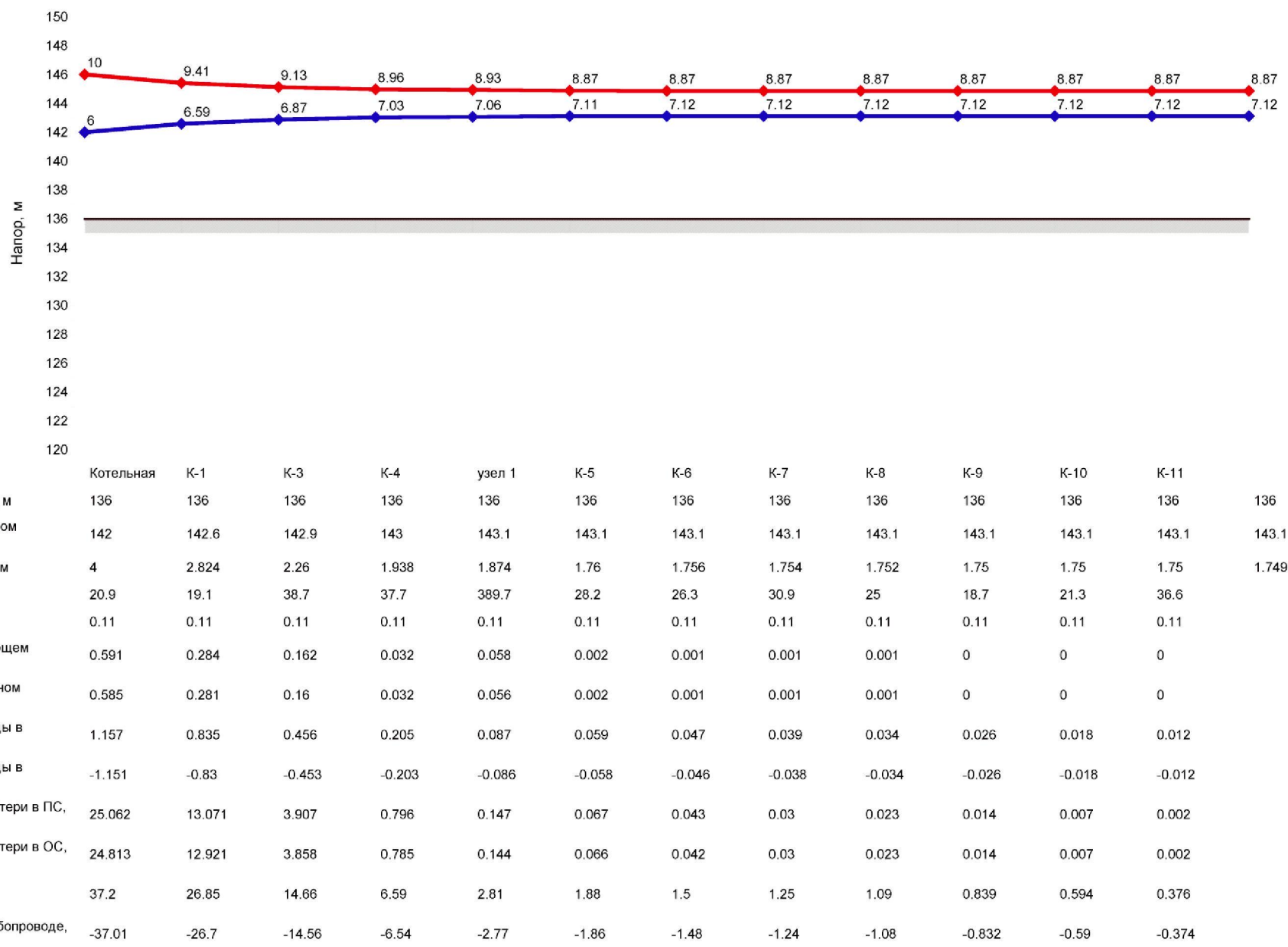
График от котельной до ул.Зеленая, 16
