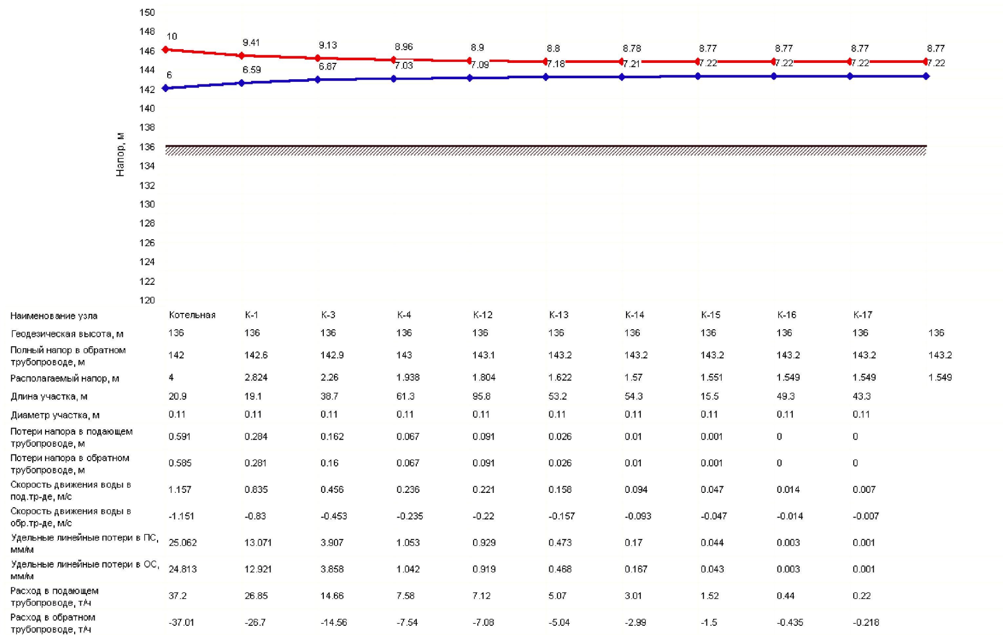
График от котельной до ул. Центральной,3
