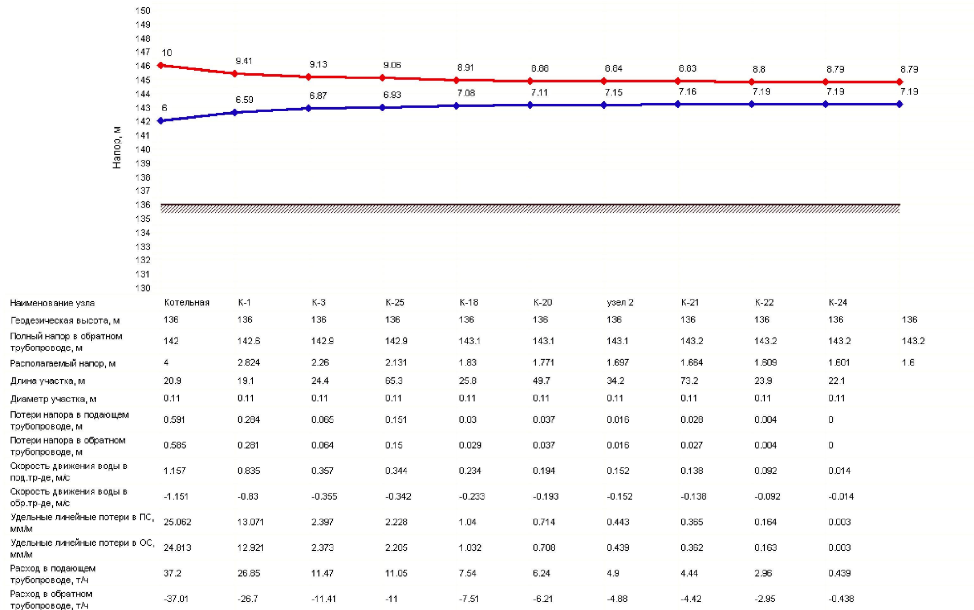
График от котельной до ул.Молодежная, 20
